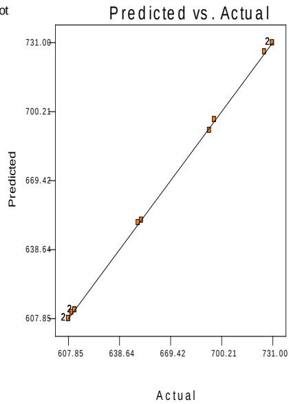
Fig. i: Tensile strength
