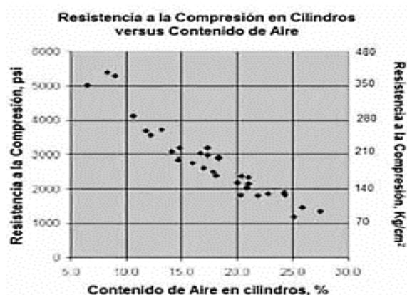
Figura 1: Gráfico de la resistencia a la compresión versus contenido de aire en especímenes de concreto permeable
