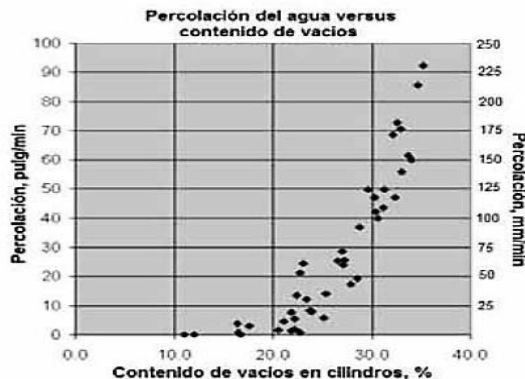
Figura 3: Gráfica de percolación versus contenido de vacíos en cilindros
