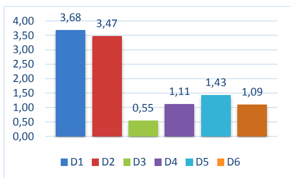
Figura 8: Permeabilidad obtenida (mm/s)
