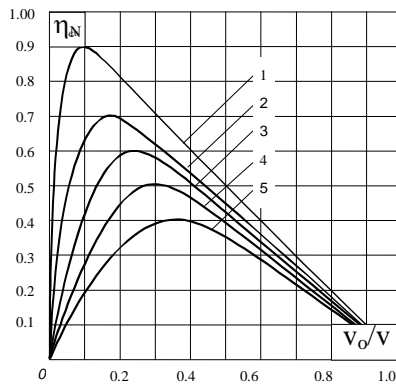
Рис.5 Обобщенная зависимость КПД ракетных двигателей от скорости полета 1,2,3,4,5 - R_{уд} / v_{в} = 1,0; 0,5; 0,2; 0,15; 0,1 .
